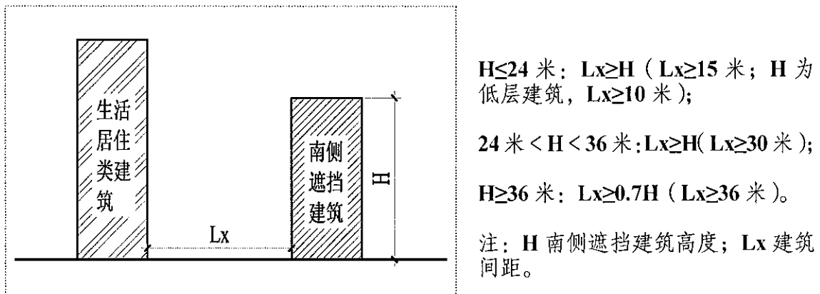
建筑间距控制示意图
